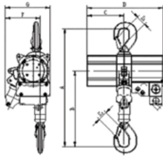
PROFI 0.25Ti - 2Ti
