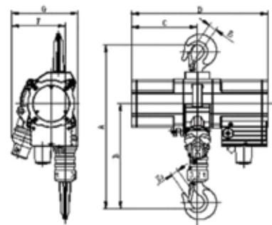
PROFI 3Ti / 20Ti
