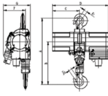
PROFI 1.5Ti - 3Ti/2
