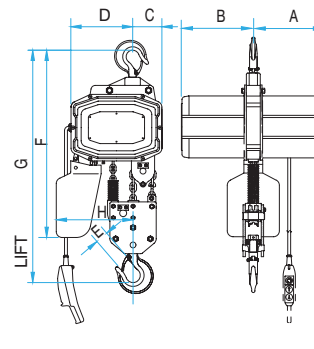
3,000kg - Triple Fall
