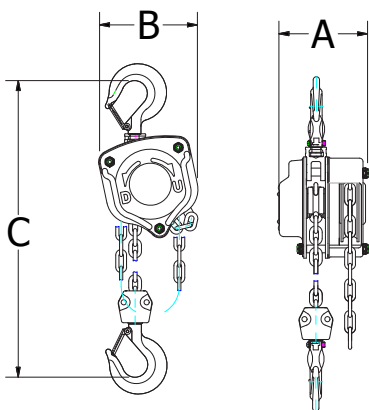
500 kg, 1 Tonne & 2 Tonne
